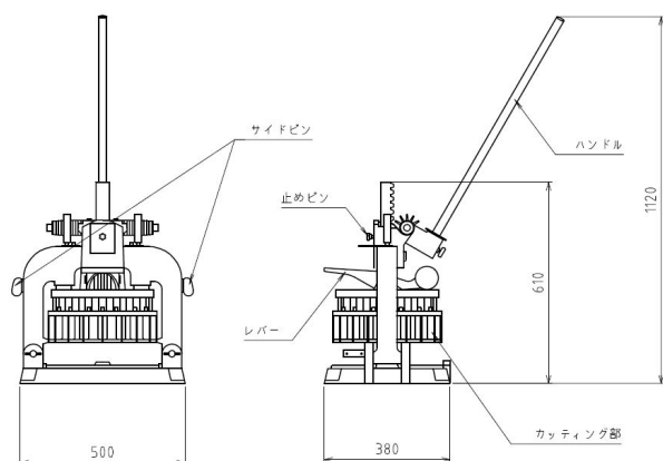
外形寸法図 (HD36)
