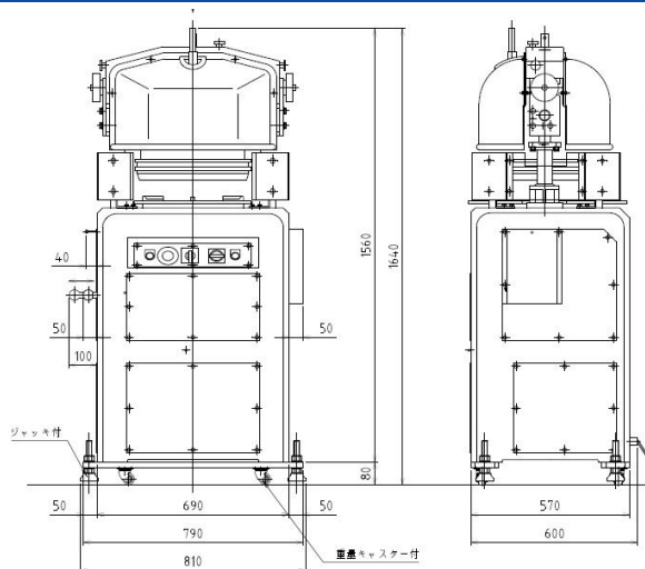
外形寸法図 (DR30B)
