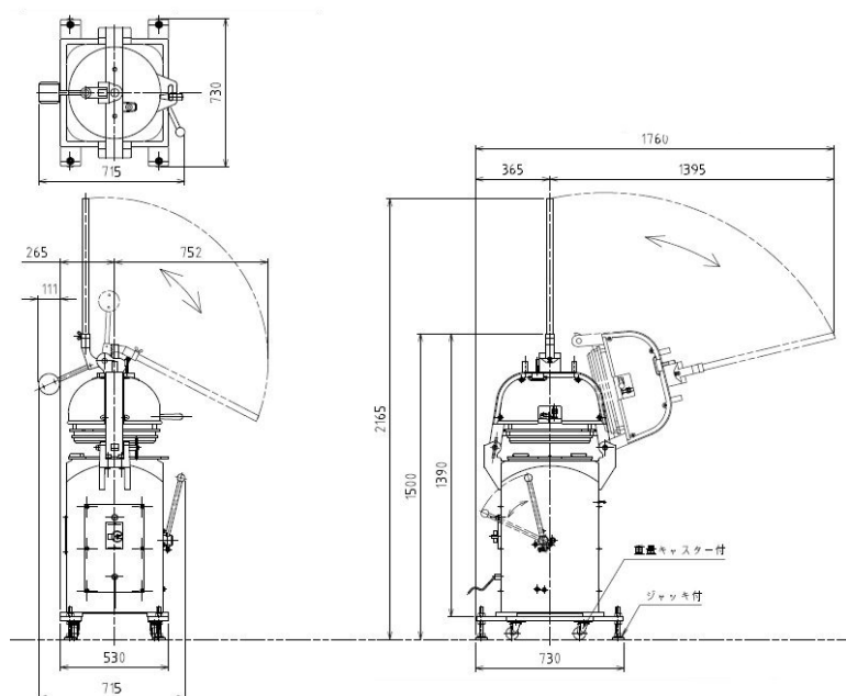
外形寸法図 (HD36)
